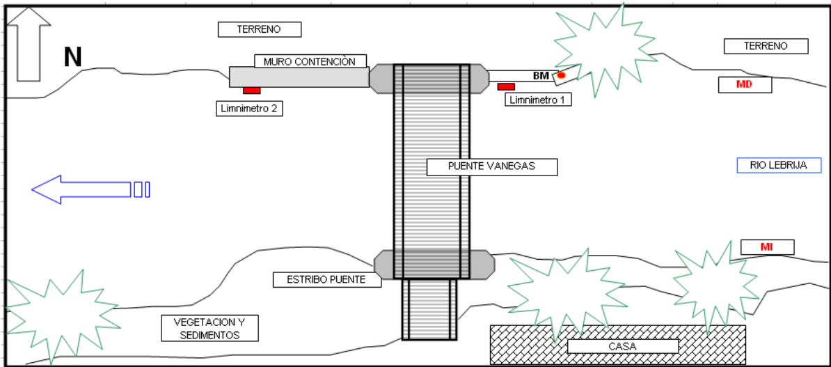
GRAFICO 36. Distribución de los limnímetros en la estación limnigráfica Vanegas municipio de Rionegro.
