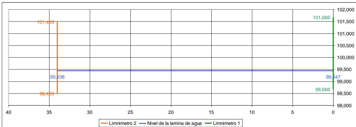
GRAFICO 37. Vista frontal del "perfil de la sección de aforo" de la estación Vanegas
